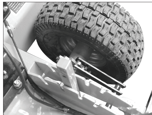
Geblocktes Laufrad mit der Fallklinke bei Frästiefeneinstellungen von 1 - 4 (MIN. - MAX.).
