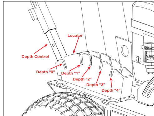
Frästiefeneinstellung
