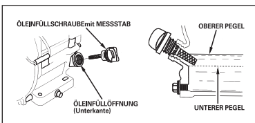
Öleinfüllschraube
