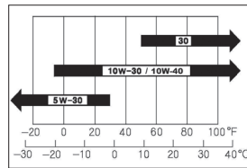
Motorenöl
