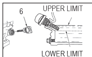
Motoröl-Einfüllschraube
