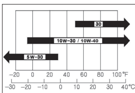
Motorenöl
